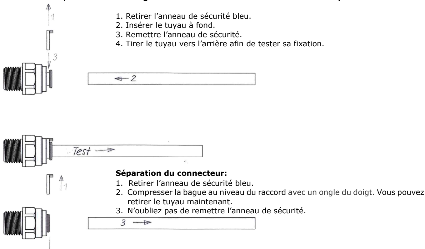
Schéma 1: Connexion des tuyaux
